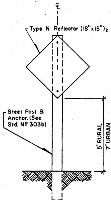
ELEVATION
